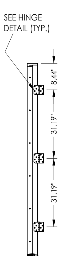
HINGE JAMB
